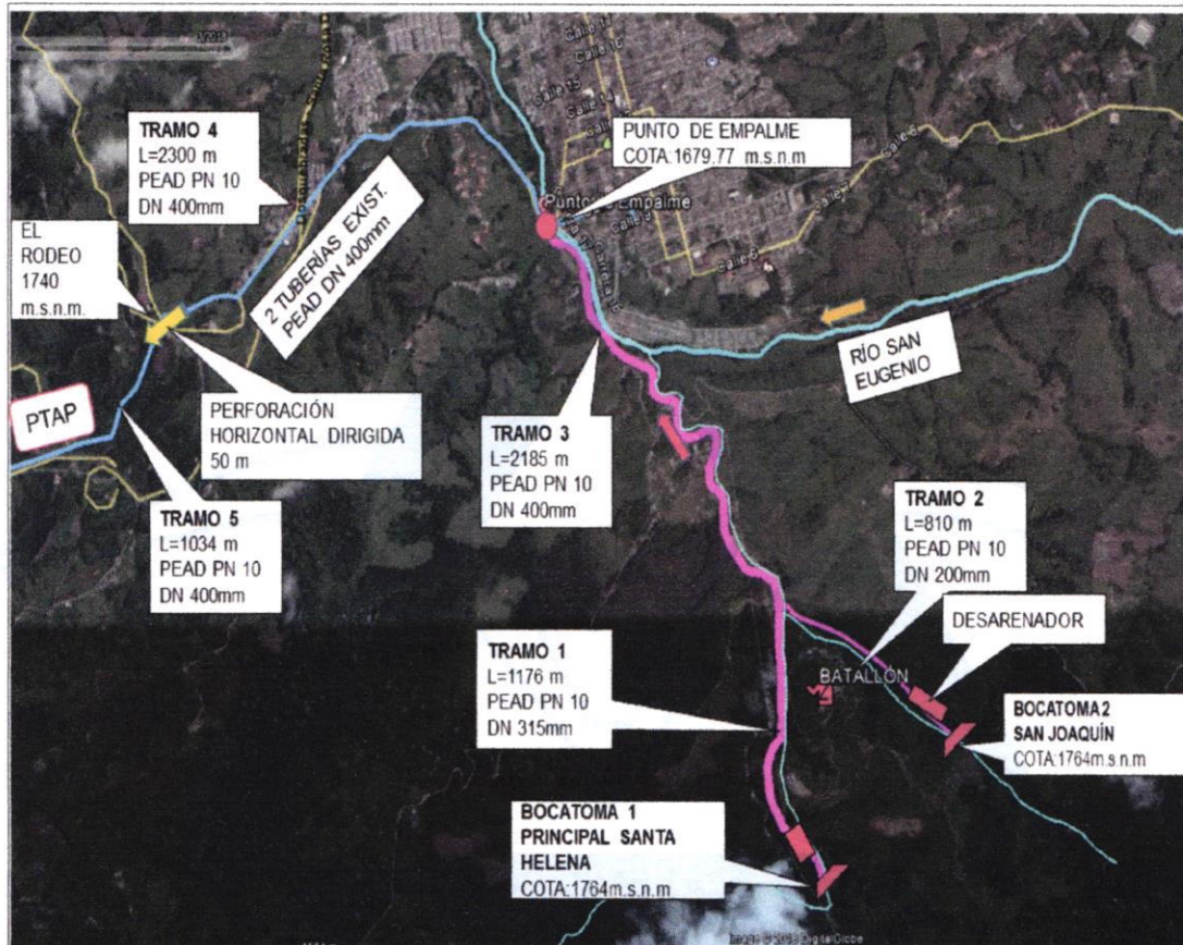
Tramo aducciones
