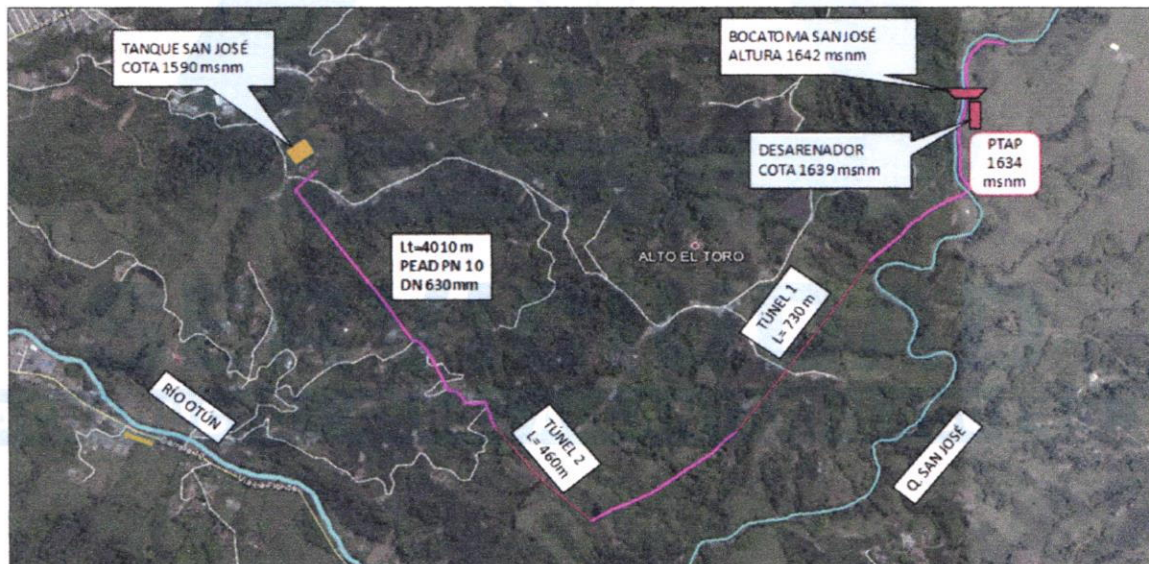
Tramo conducción
